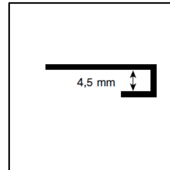
Төгсгөлийн С-профил 2800 mm
